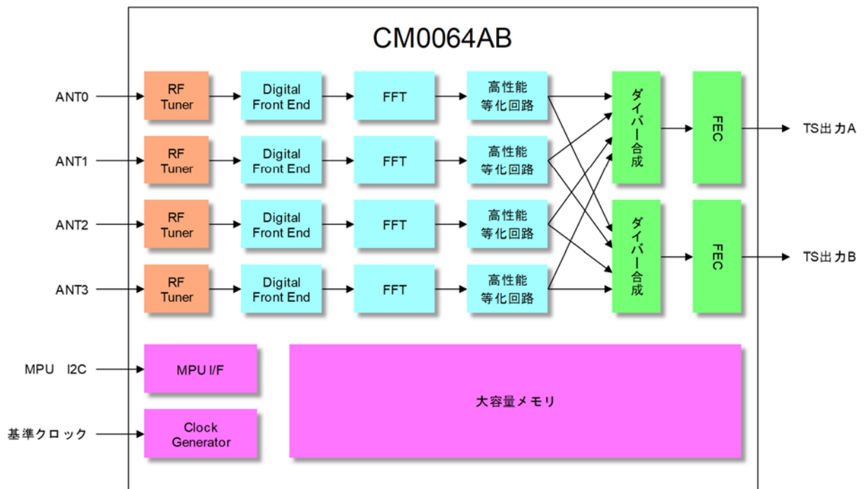
Fig. 2-1 : ブロック図
